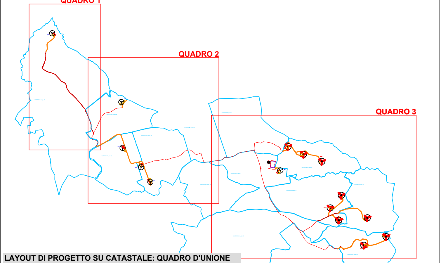
LAYOUT DI PROGETTO SU CATASTALE: QUADRO D'UNIONE
