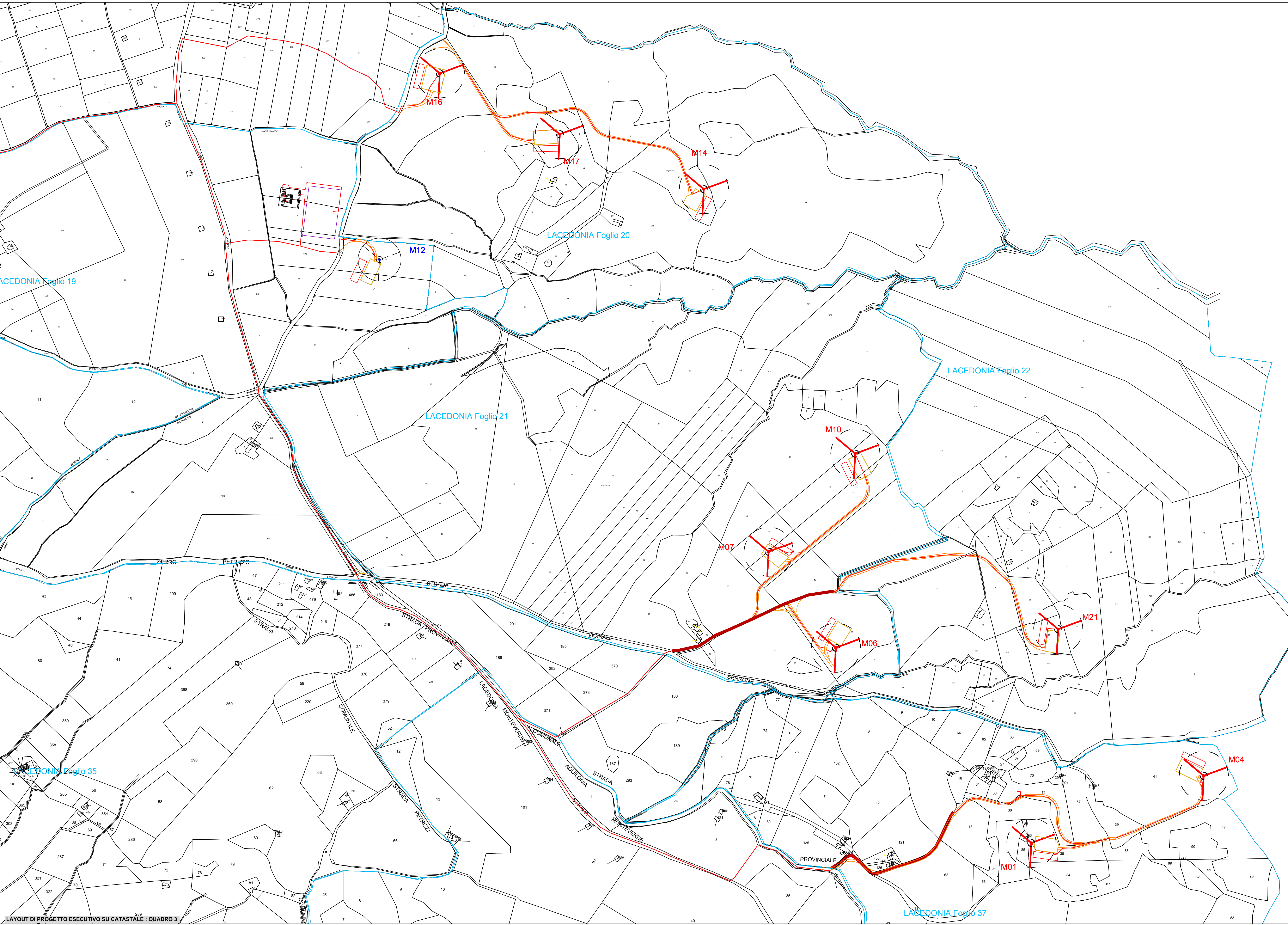
LAYOUT DI PROGETTO ESECUTIVO SU CATASTALE : QUADRO 3
