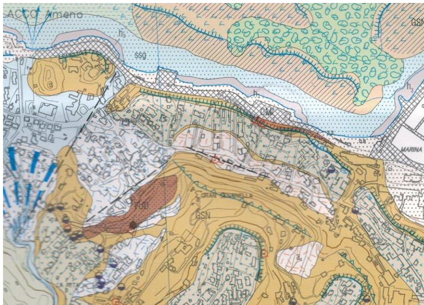
Fig. 2.c.1. stralcio della carta geologica C.A.R.G.
