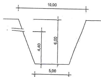
SEZIONE PUNTO DI SCARICO
