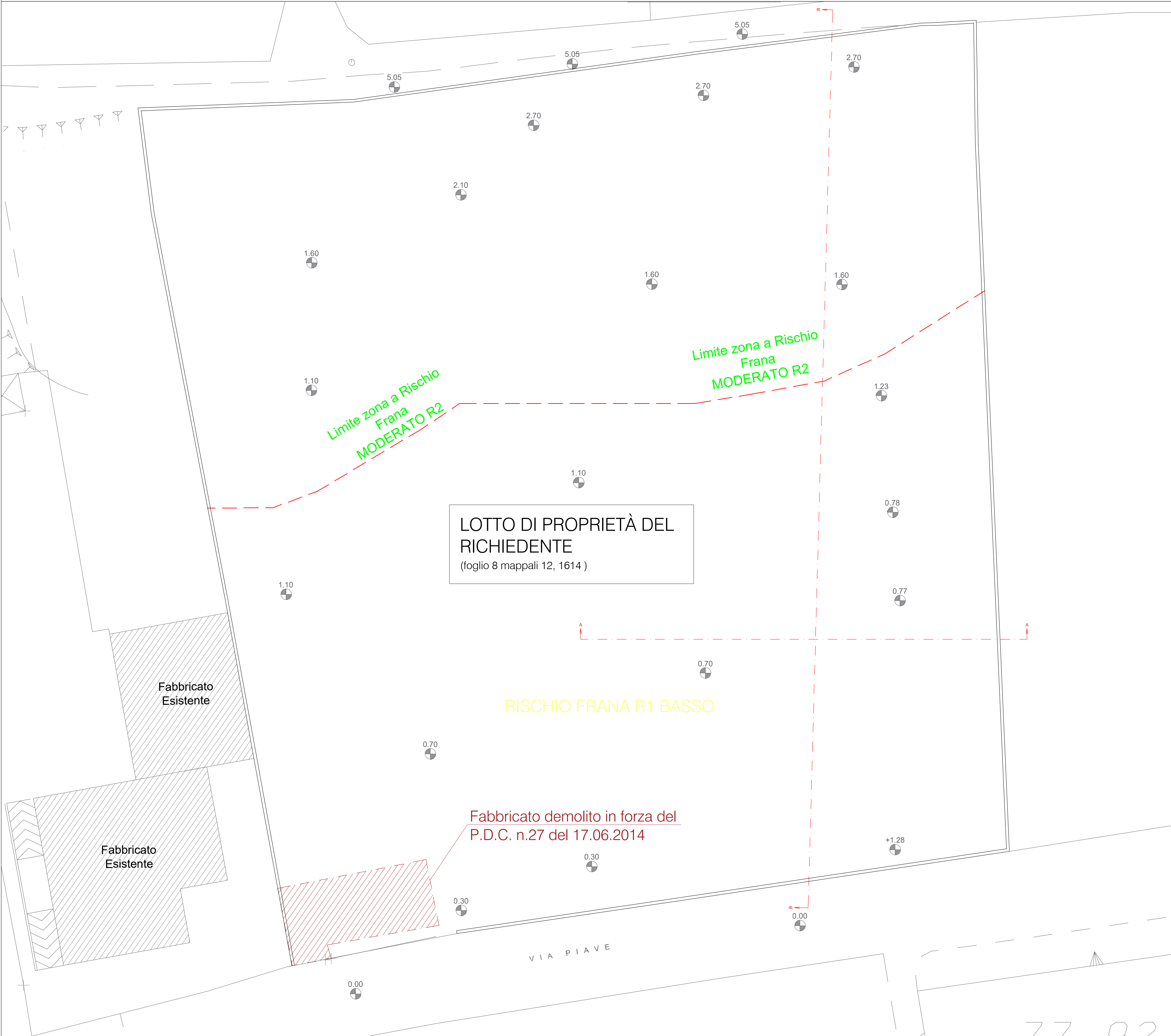
STATO DI FATTO _ PLANIMETRIA GENERALE _ SCALA 1:200
