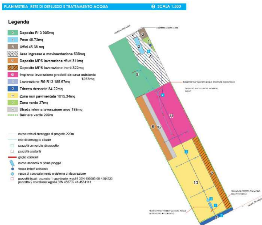
Figura 3 – Planimetria rete di flusso e trattamento acque.
