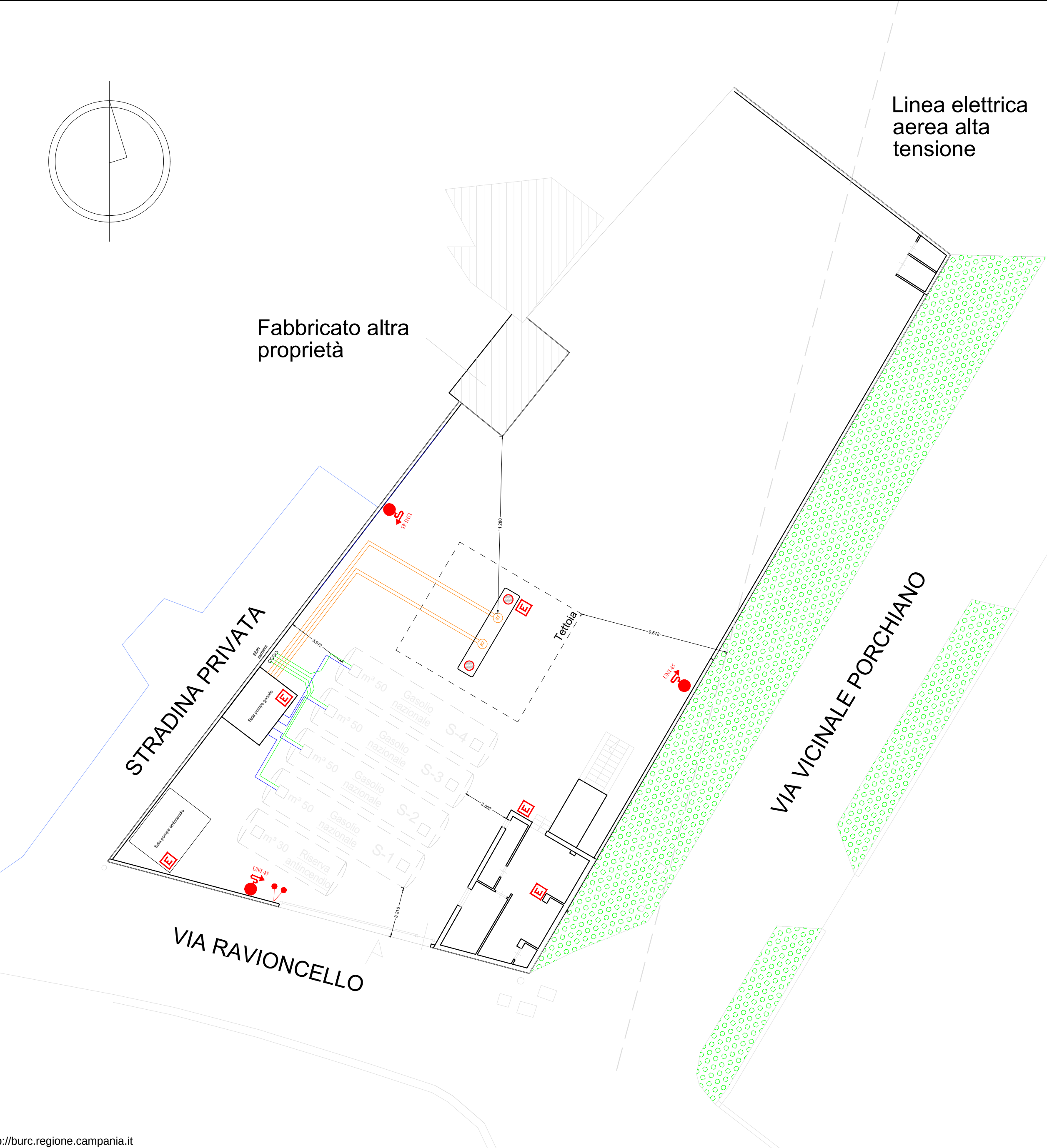
PLANIMETRIA CON LAYOUT- scala 1:200
