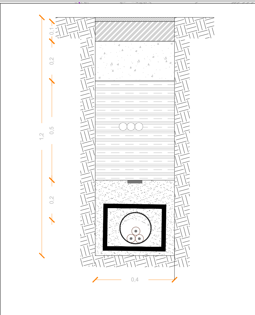
Particolare sezione scavo su strada asfaltata pubblica N. C. d. S. scala 1:5
