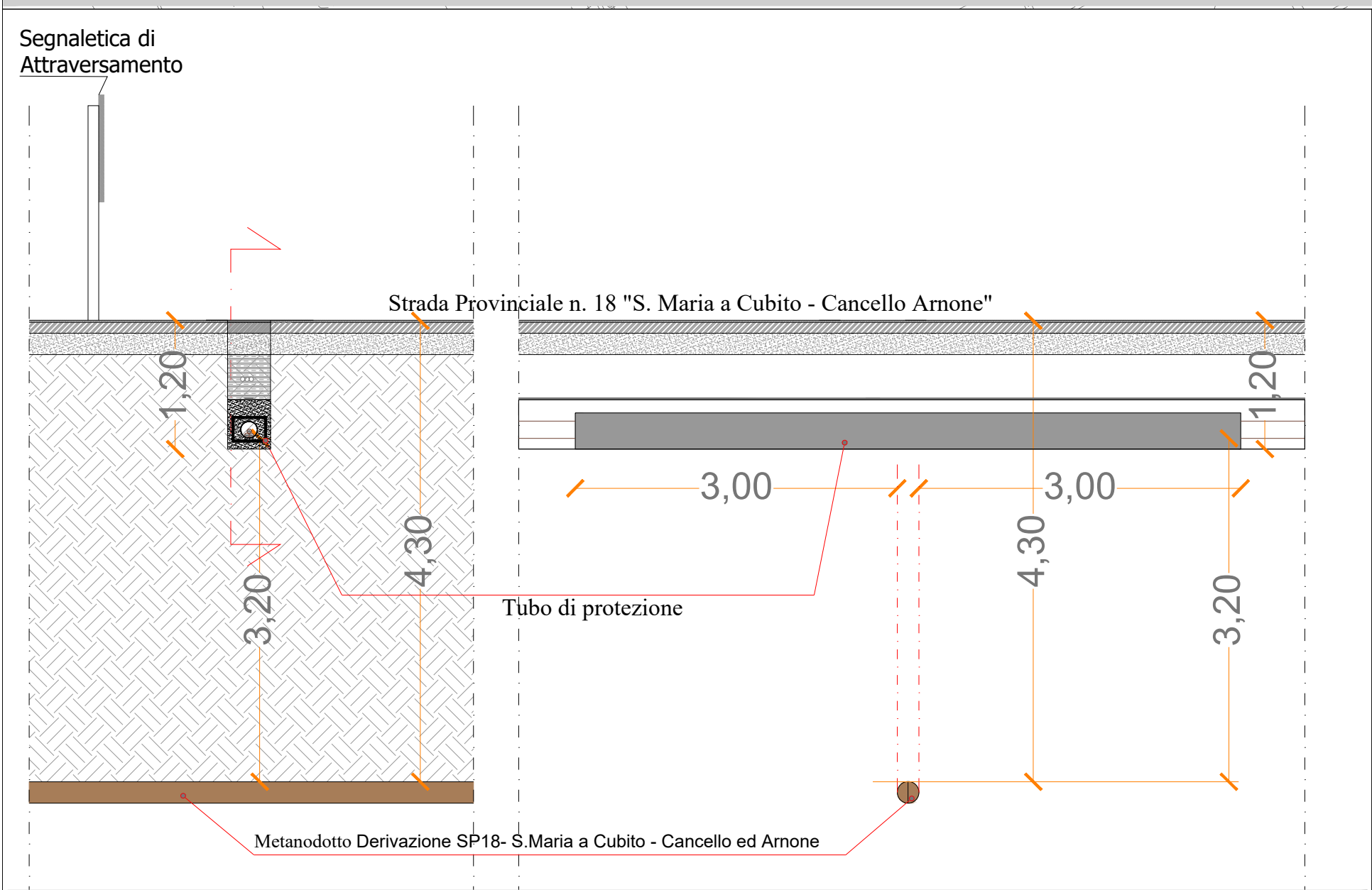
Sezione attraversamento gasdotto SNAM Scala 1:20
