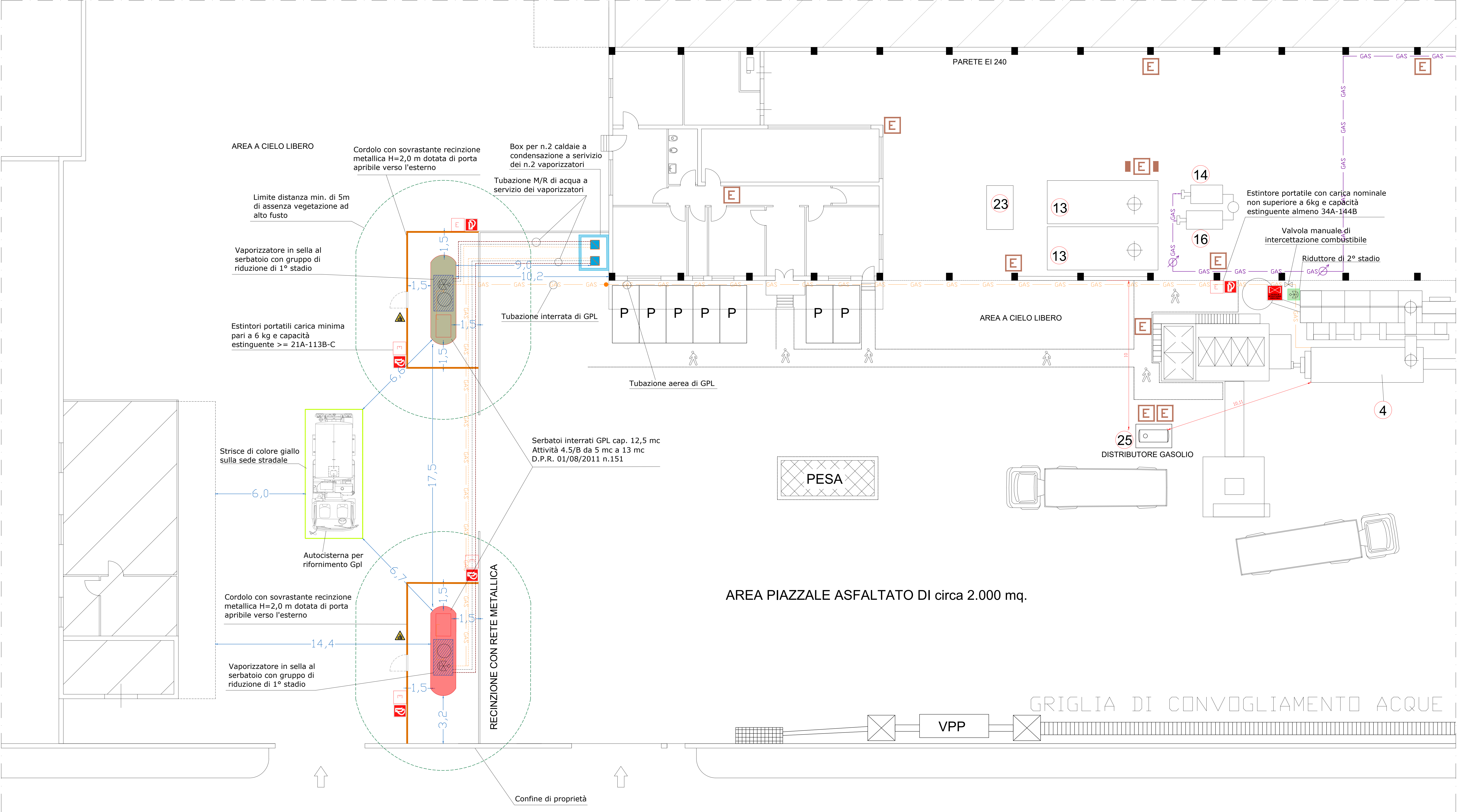
Planimetria dettaglio - Layout serbatoi costituenti il deposito di oli minerali - Scala 1:100
