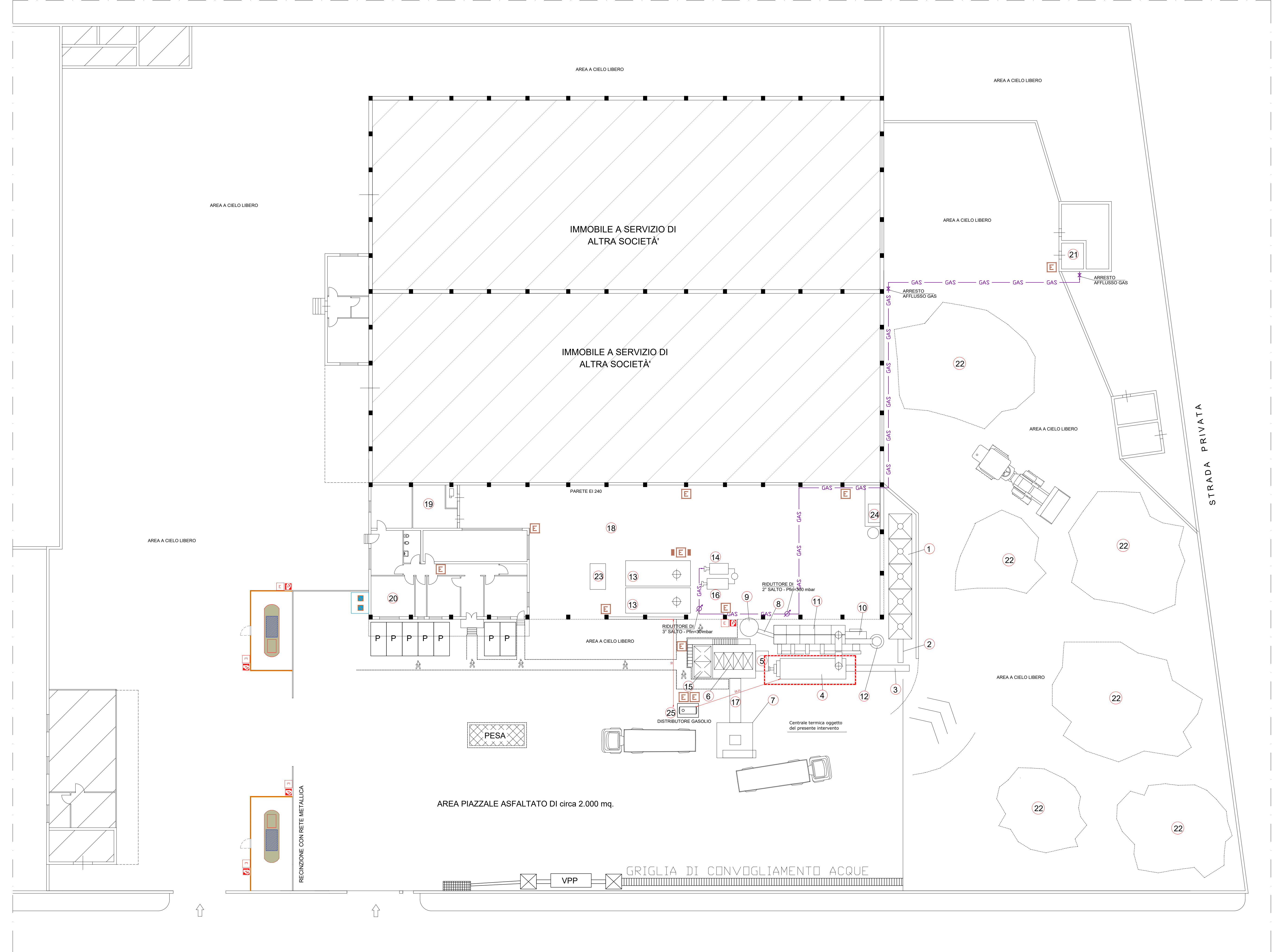
Planimetria generale del sito produttivo - Scala 1:200
