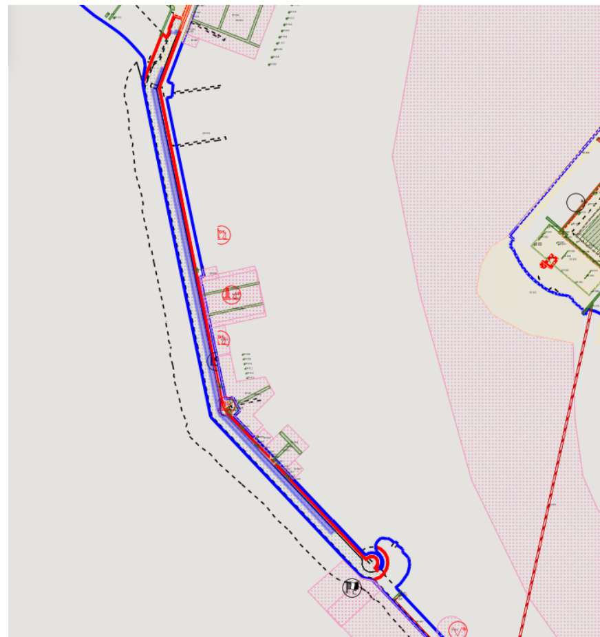
- Planimetria di dettaglio Concessione
