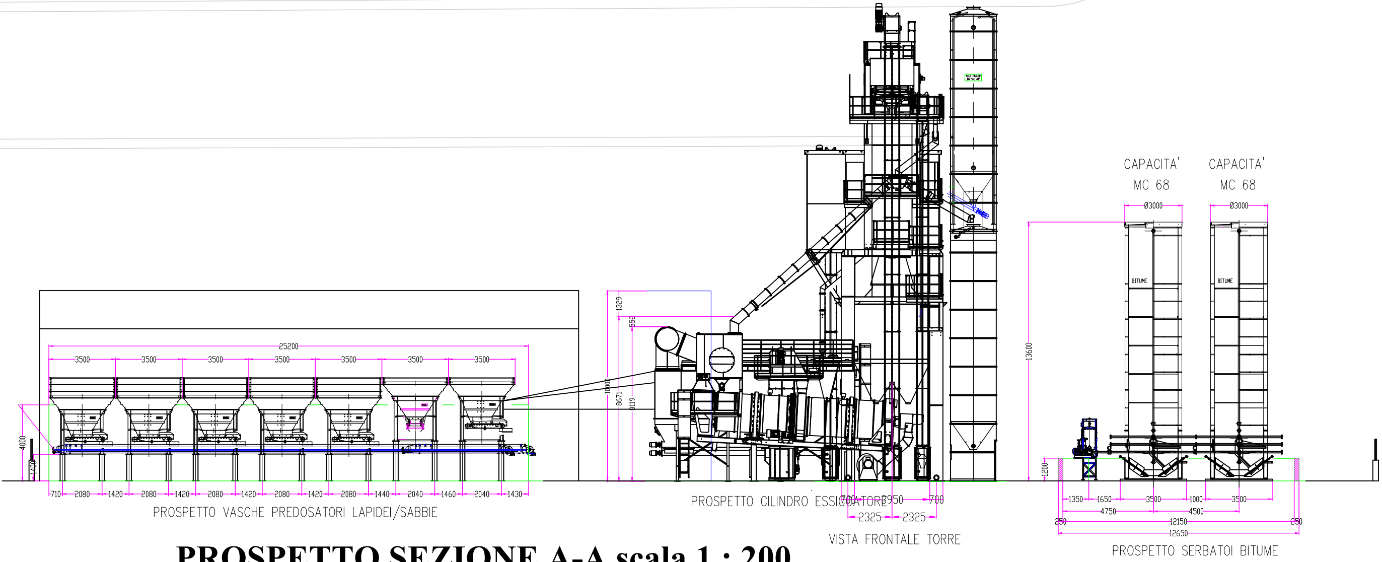
PROSPETTO SEZIONE A-A scala 1 : 200
