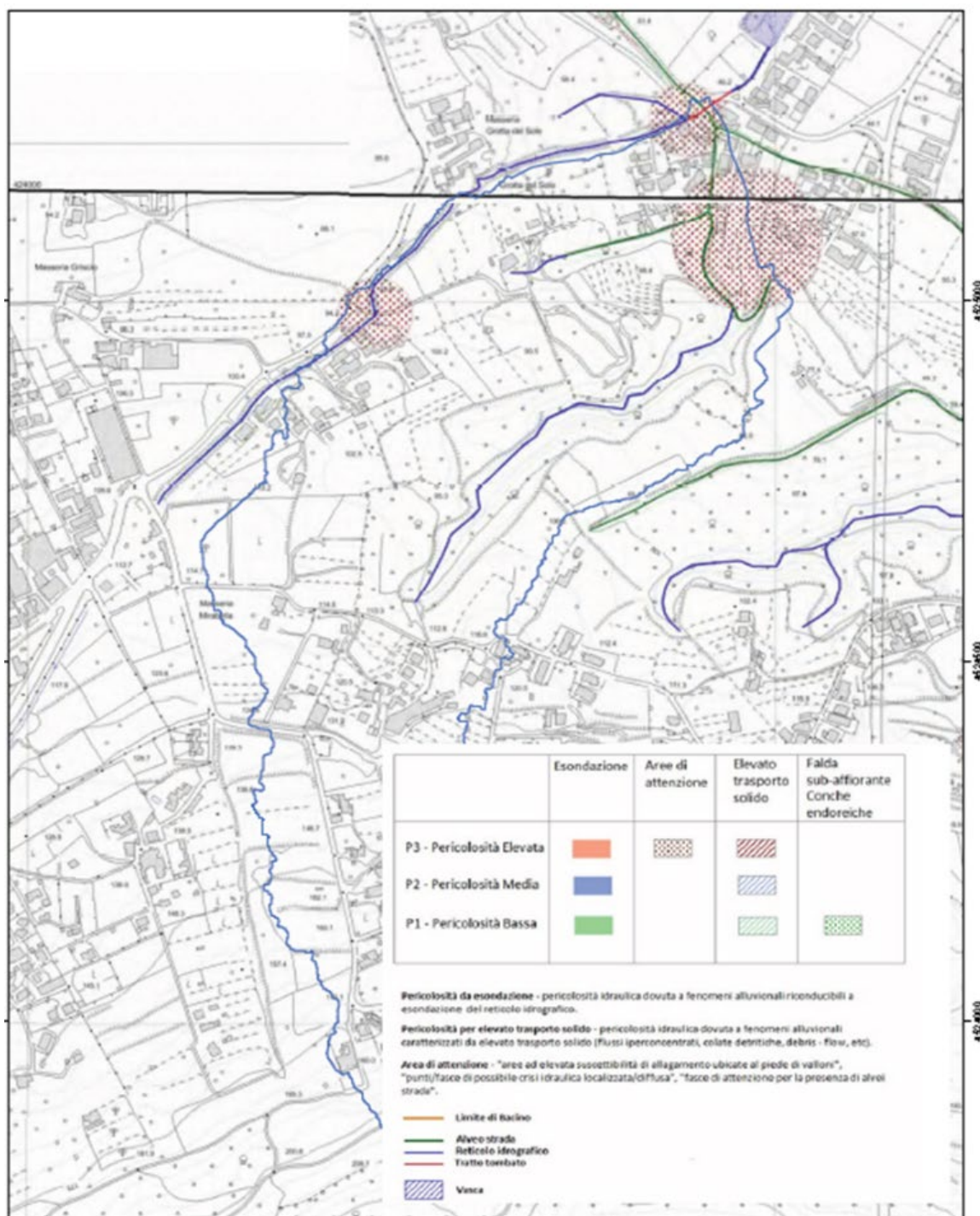
Comune di Pozzuoli (NA) - Località Grotta del Sole - Piano Stralcio di Assetto idrogeologico dell'ex AdB Campania Centrale - Stralcio mappa della pericolosità idraulica vigente - tavv.447103P e 447101P.
