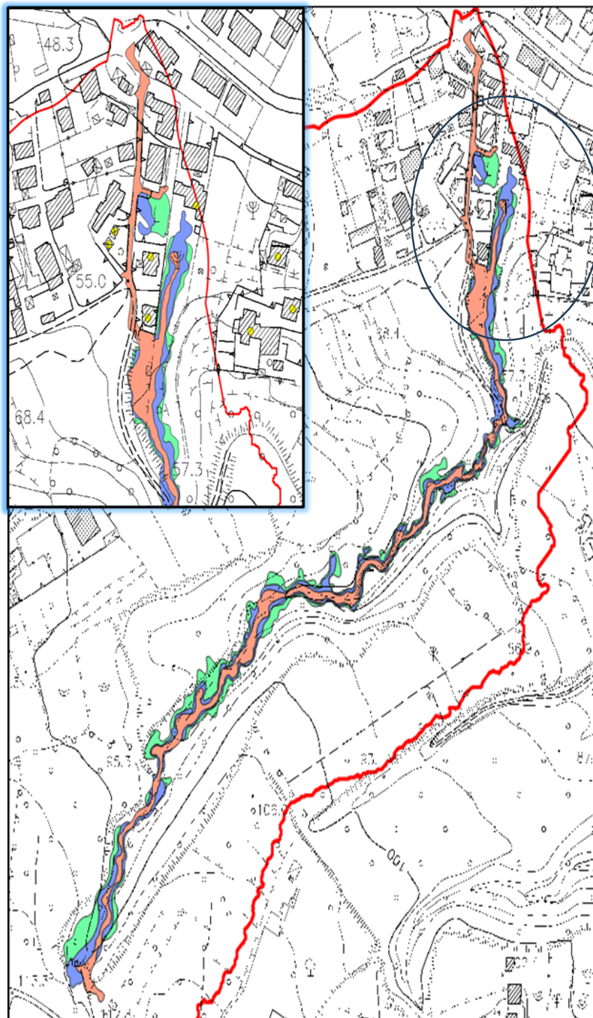
Comune di Pozzuoli (NA) - Località Grotta del Sole - Piano Stralcio di Assetto idrogeologico dell'ex AdB Campania Centrale - Stralcio mappa della pericolosità idraulica proposta tavv. 447103P e 447101P;
