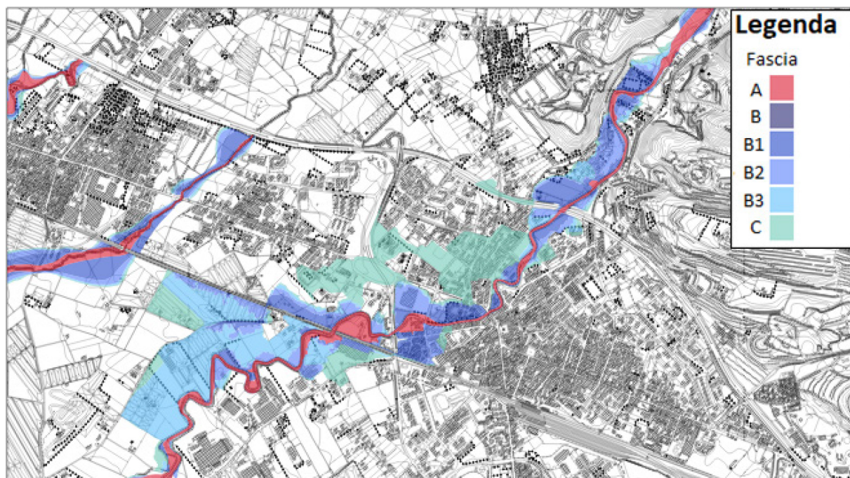
Comune di Battipaglia (SA) – fiume Tusciano – Piano Stralcio di Assetto idrogeologico dell'ex Autorità di Bacino Regionale Destra Sele – Stralcio mappa delle fasce fluviali proposta (tavv. I_FFI_467161 – I_FFI_467162 – I_FFI_467163)
