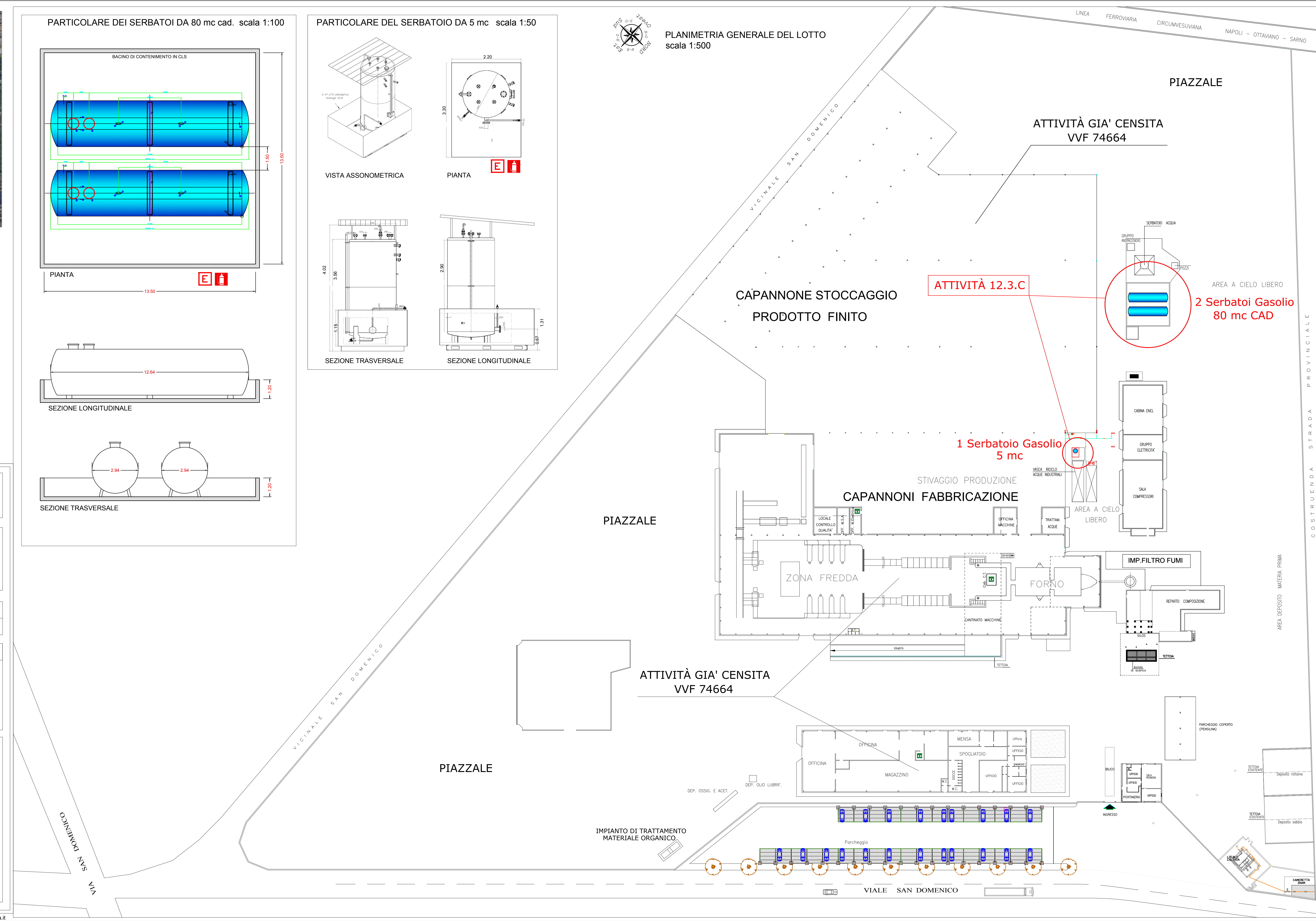
STRALCIO PLANIMETRICO scala 1:200
