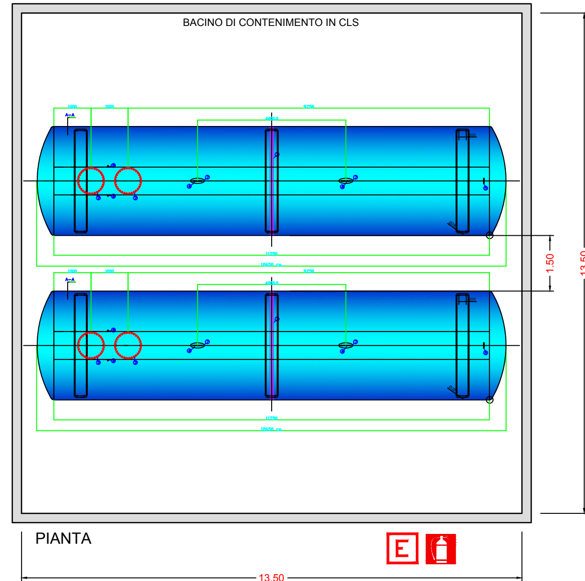
PARTICOLARE DEI SERBATOI DA 80 mc cad. scala 1:100
