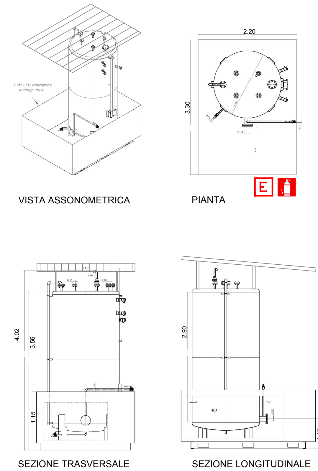
PARTICOLARE DEL SERBATOIO DA 5 mc scala 1:50
