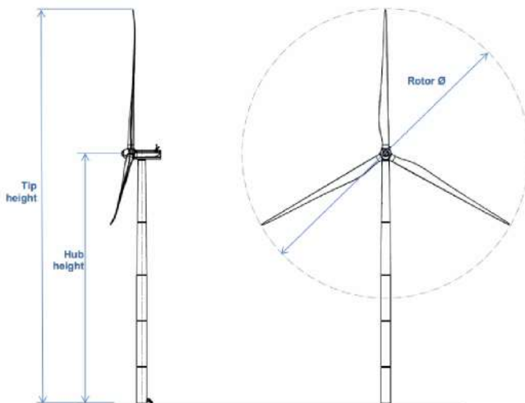
Figura 22 – Caratteristiche geometriche aerogeneratore di progetto
