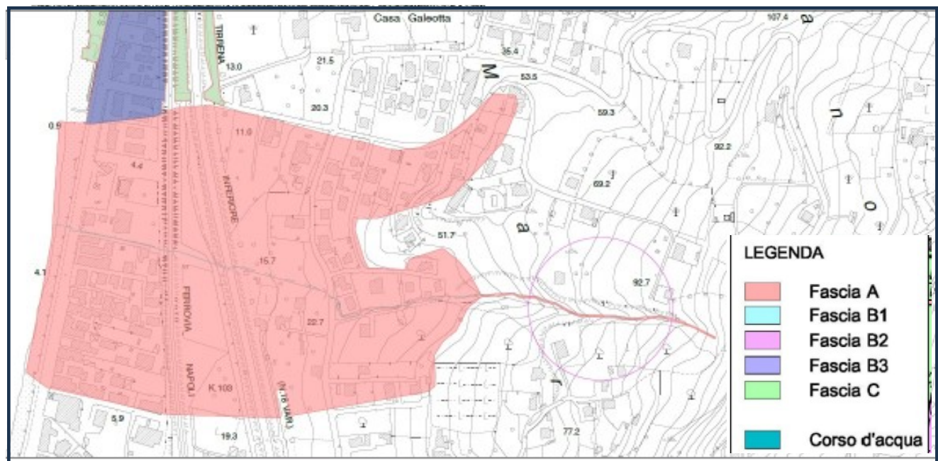
Comune di Agropoli (SA) – Torrente Galliano – Piano Stralcio di Assetto idrogeologico dell'ex Autorità di Bacino Regionale Campania Sud e Interregionale del Sele (UoM - Sx Sele) – Stralcio Mappa delle Fasce fluviali approvata - Torrente Galeotta tav. 1/1.
