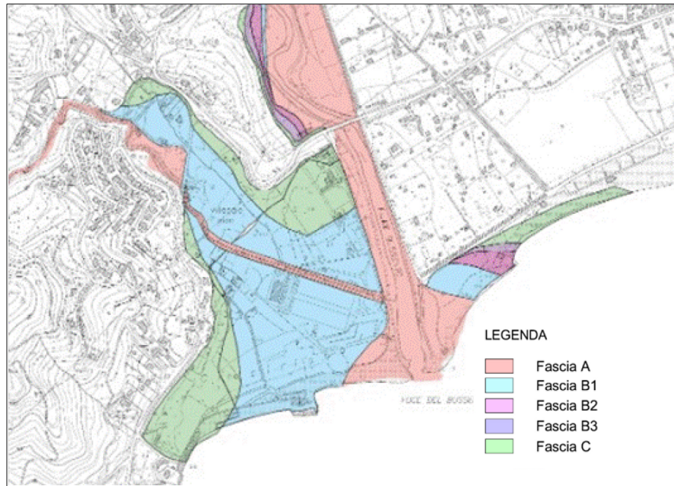
Comune di Santa Marina (SA) – Vallone Aria della Serra – Piano Stralcio di Assetto idrogeologico dell'ex Autorità di Bacino Regionale Campania Sud e Interregionale del Sele (UoM - Sx Sele) – Stralcio Mappa Fiume Bussento - Fasce Tavola 5/5, vigente
