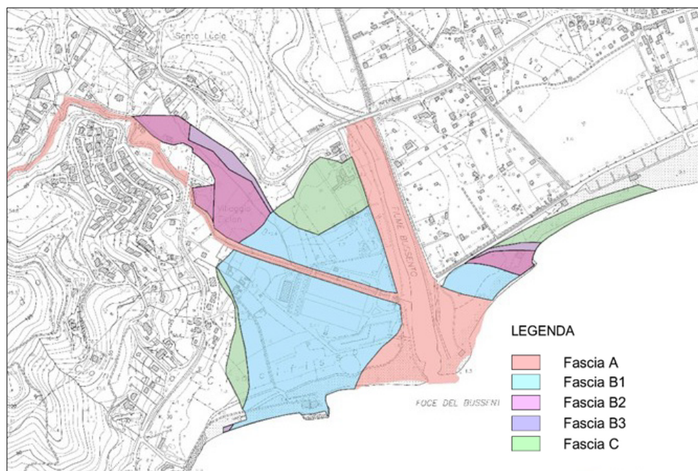
Comune di Santa Marina (SA) – Vallone Aria della Serra – Piano Stralcio di Assetto idrogeologico dell'ex Autorità di Bacino Regionale Campania Sud e Interregionale del Sele (UoM - Sx Sele) – Stralcio Mappa Fiume Bussento - Fasce Tavola 5/5, proposta
