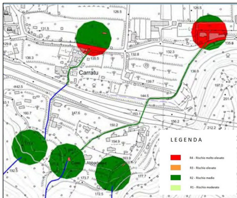
Comune di Mercato San Severino (SA) – Via Carratù – Piano Stralcio di Assetto idrogeologico dell'ex Autorità di Bacino Regionale Campania Centrale – Stralcio Mappa del Rischio idraulico vigente Tavola RI-467012.
