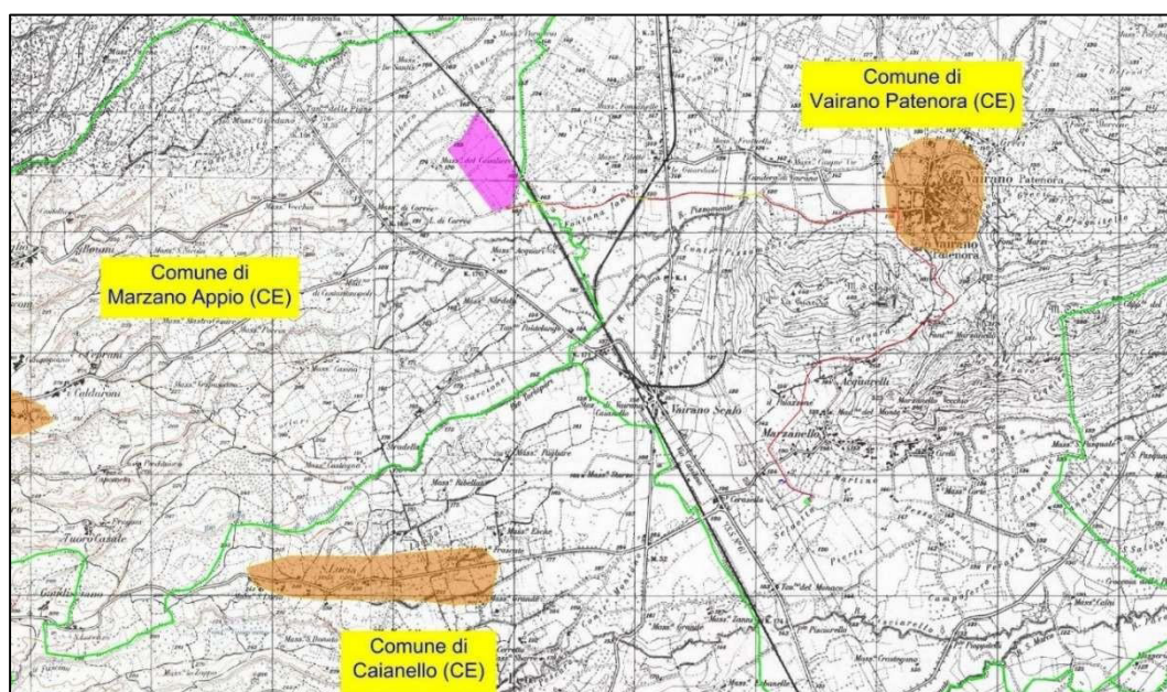
Figura 3 - Inquadramento dell’area di impianto e delle opere di connessione su IGM (Rif. FV.MRA01.PD.B.01)
