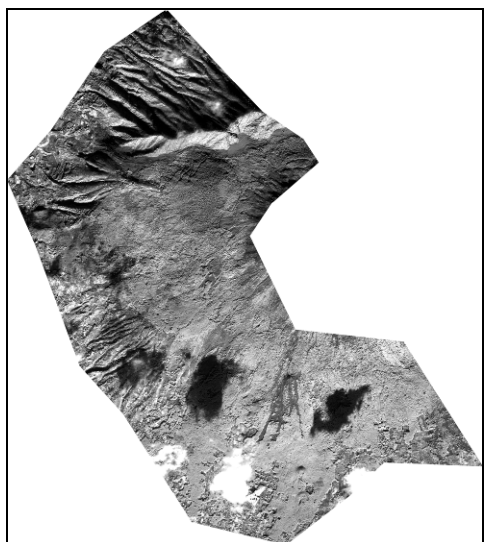
Fig. 128: Immagine satellitare del dicembre 2007 nella banda spettrale dell'infrarosso vicino
