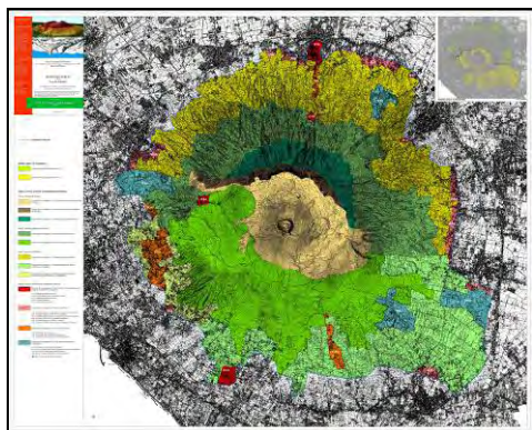
Fig. 22: Le unità elementari di paesaggio
