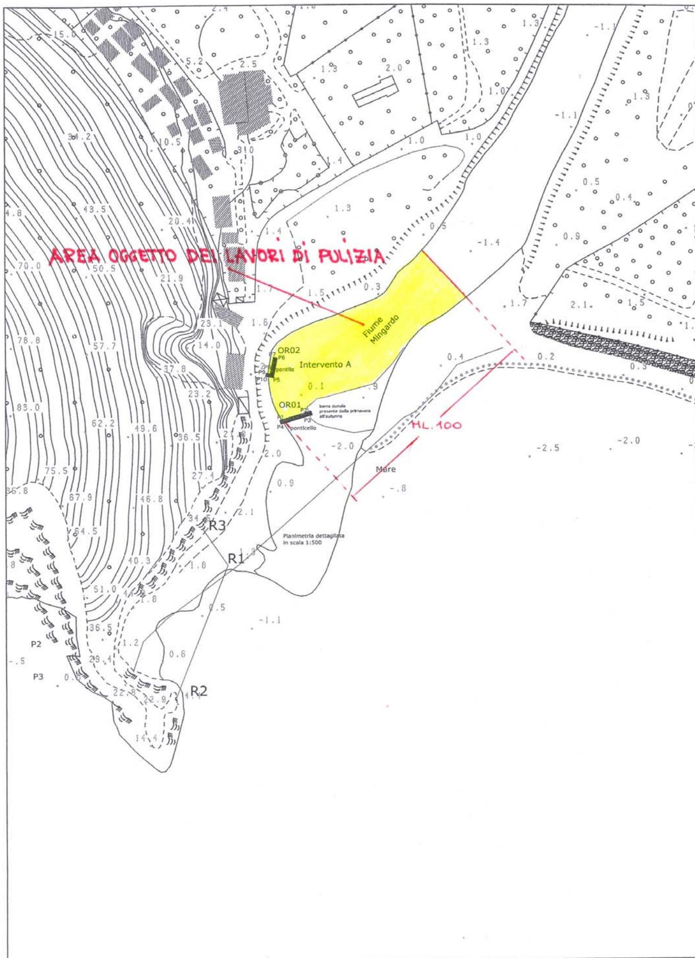
Comune di Centola Planimetria dettagliata in scala 1:2000
