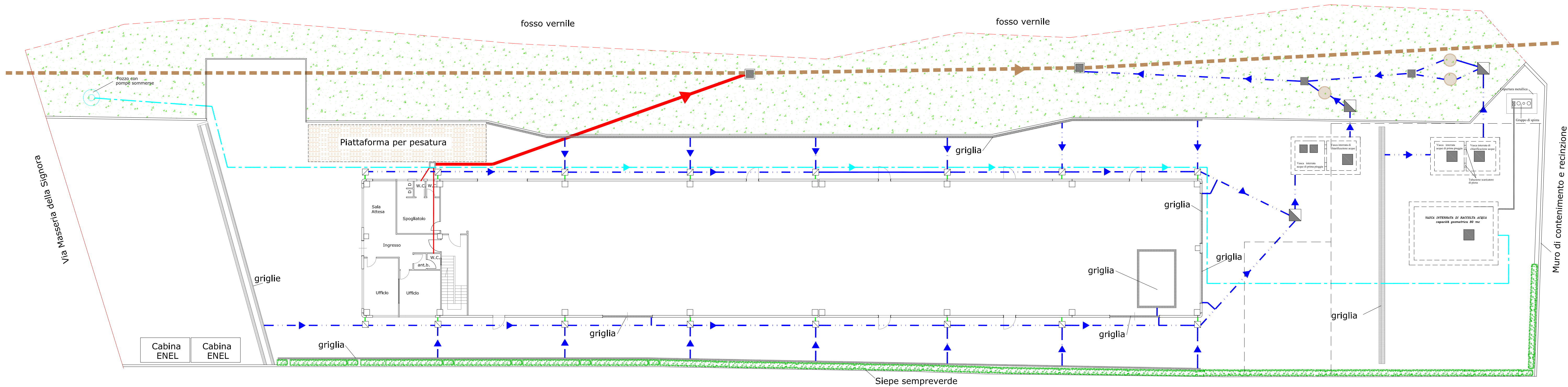
Schema vasca di prima pioggia
