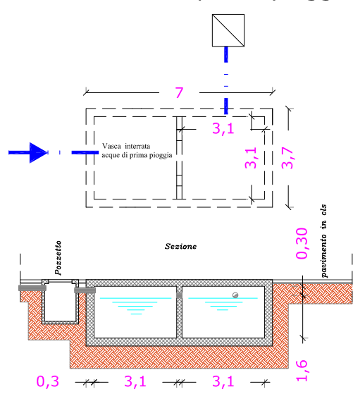
Schema vasca di prima pioggia
